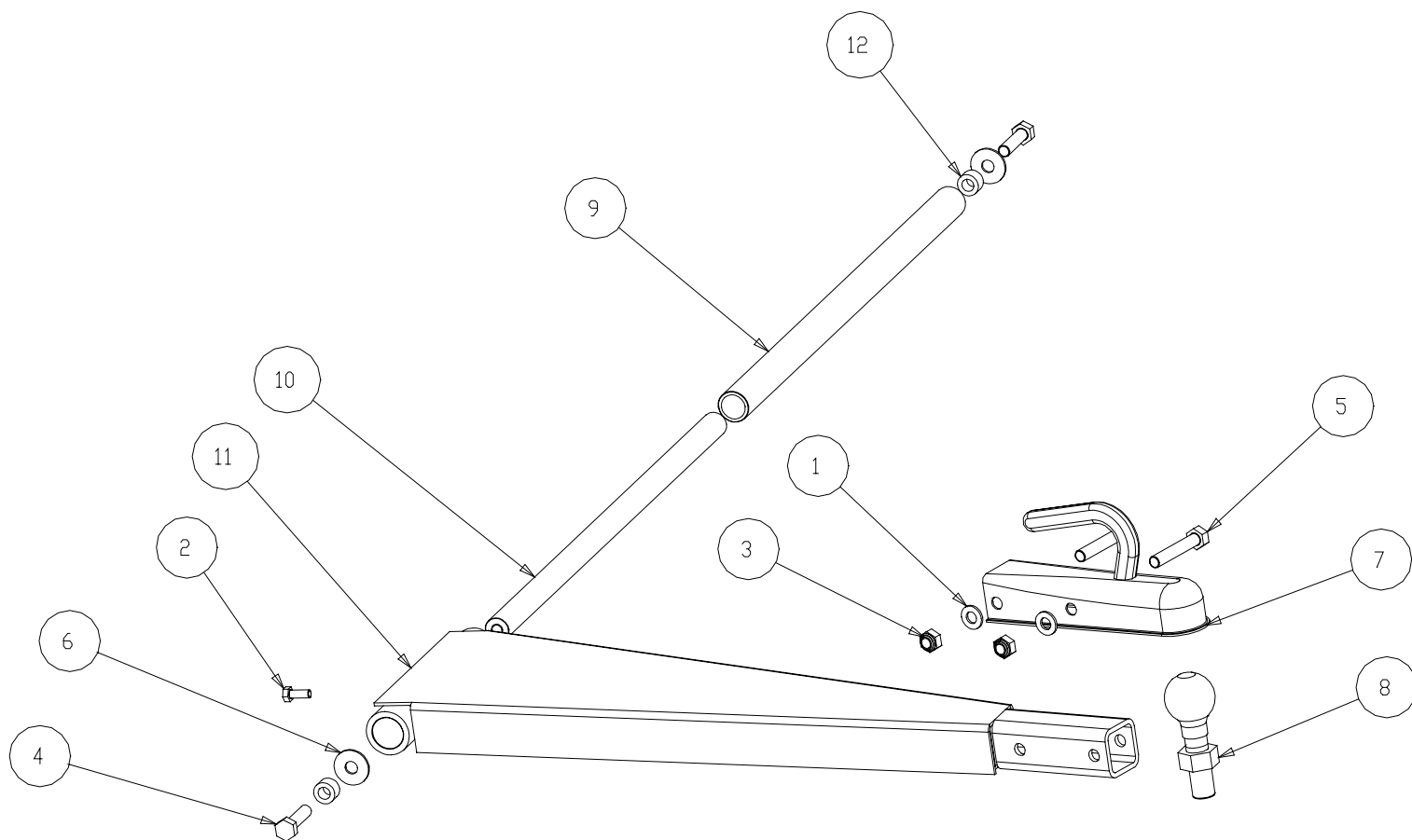
TAVOLA 3 CSP_00236- CSP_00237 Timone completo
